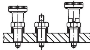
croquis 3
